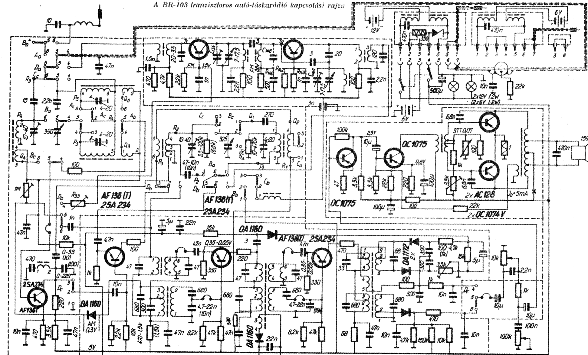
A BR-103 tranzisztoros autó-táskarádió kapcsolási rajza
