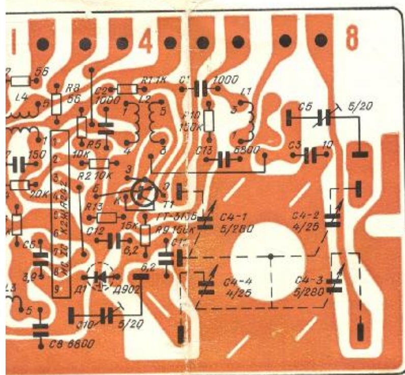
2. Схема соединений радиоэлементов на плате (приемник; блок УКВ). Connection diagram of radio components assembled on circuit board (Receiver; UKB block).
