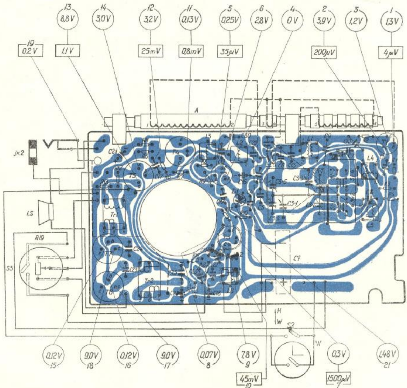
Рис. 3. Электромонтажная схема приемника Fig. 3. Wiring Diagram of Receiver
