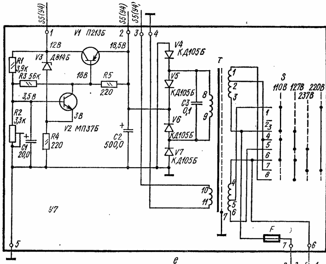
Рис. 26. Принципиальная электрическая схема приемника «Рн-га-104»:
