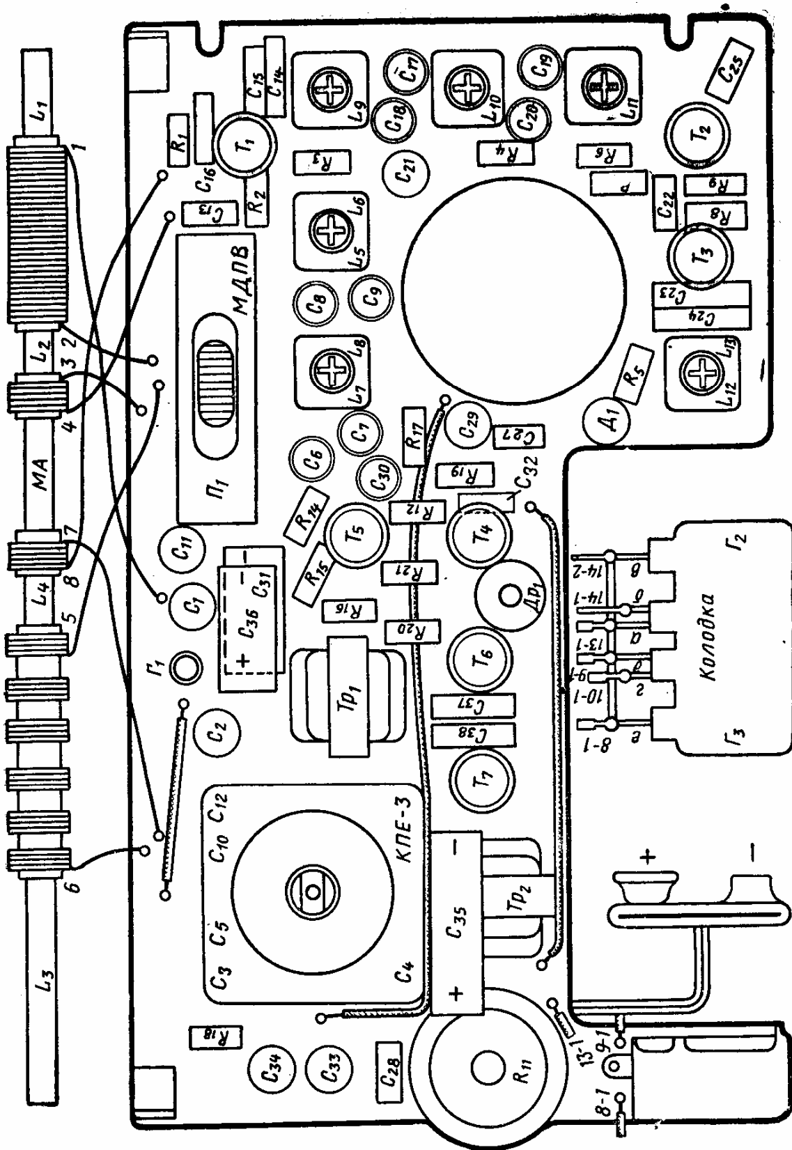
Рис. 3.41. Схема расположения узлов и деталей на печатной плате приемника «Планета».
