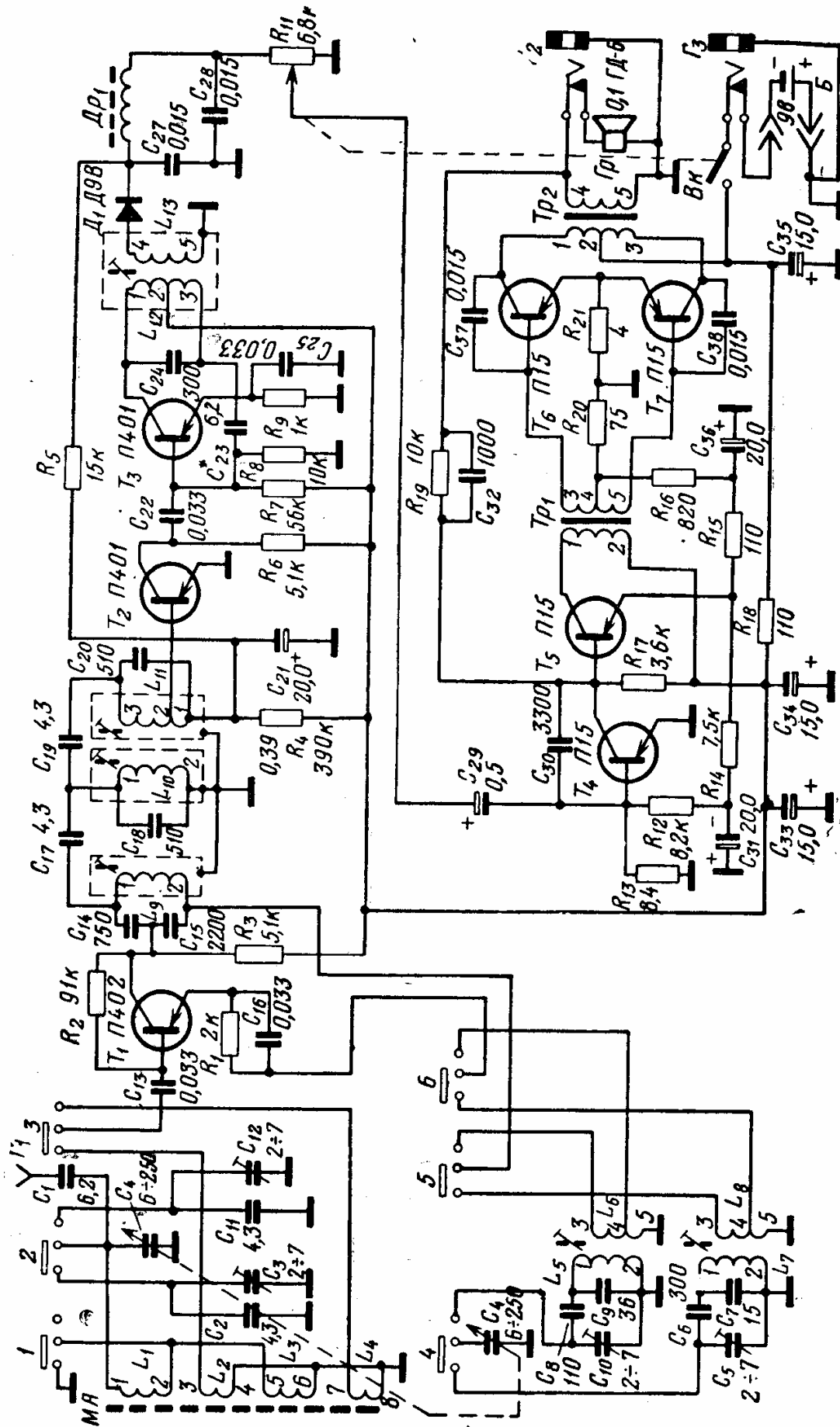
Рис. 3.39. Принципиальная схема приемника «Планета». Переключатель диапазонов установлен в положение СВ.
