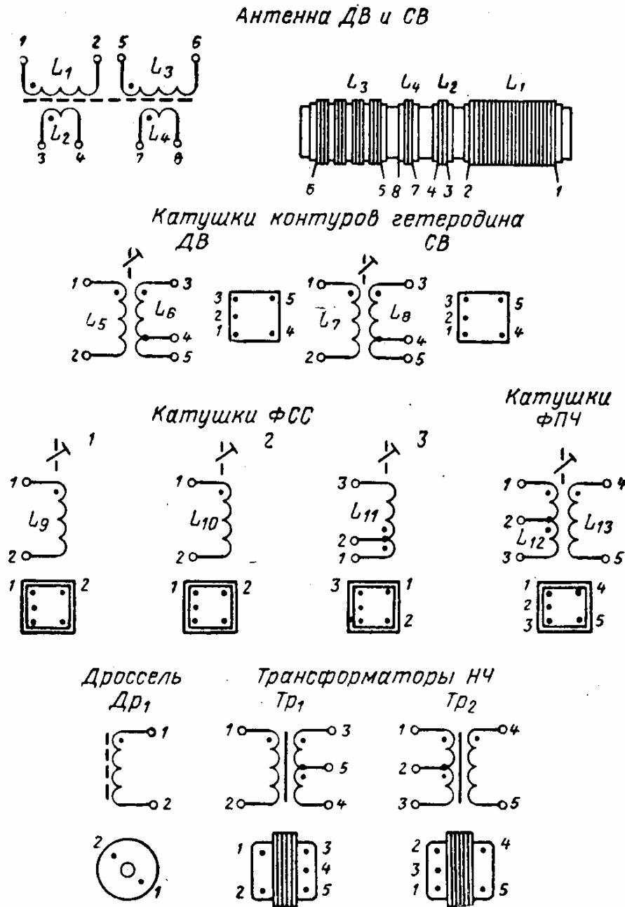
Рис. 3.42. Распайка выводов (вид снизу) катушек контуров и трансформаторов НЧ приемника «Планета».
