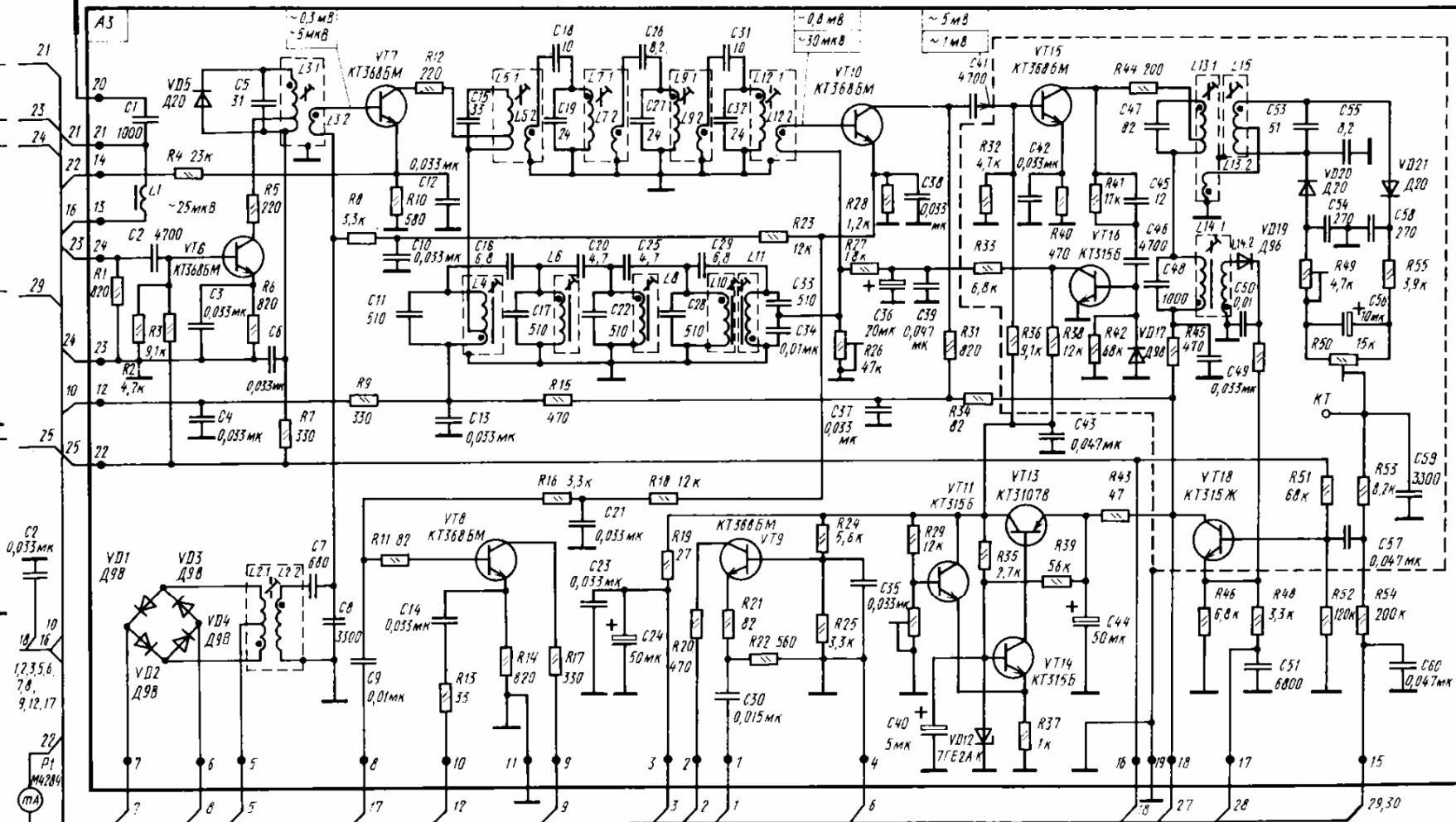
Блок РЧ-ПЧ
