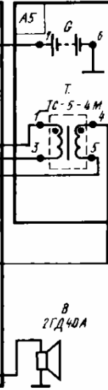
Блок питания
