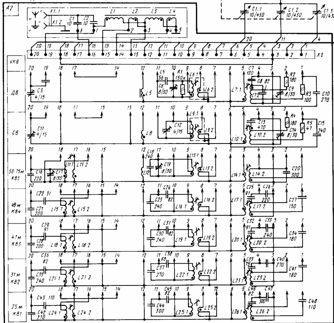
Блок КСДВ
