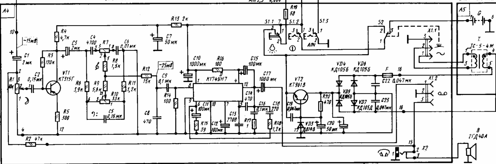
Радиоприемник ОКЕАН-214
