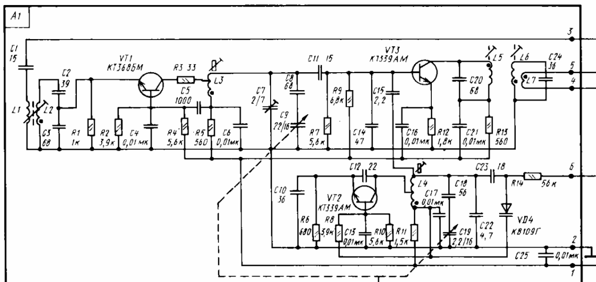
Блок КСДВ
