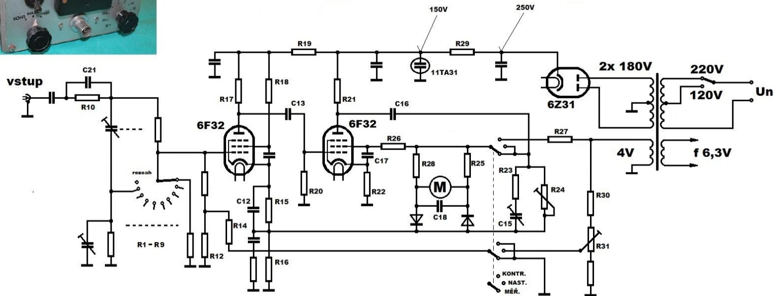
Milivoltmetr ZUŠ TESLA BRNO TM 101 Podle obvodů nakreslil Heřmánek www.csla.cz schéma v1.0
